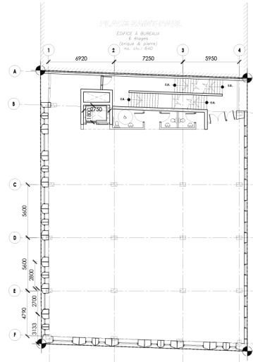
NIVEAU 2-4-6
