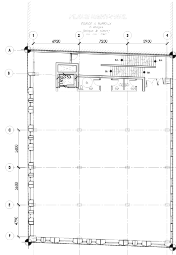
NIVEAU 3-5
